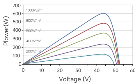
Power-Voltage(600W)
